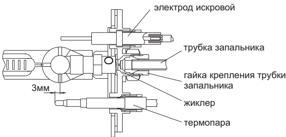
Рис. 4. Горелочное устройство КНС-2; КНС-3
