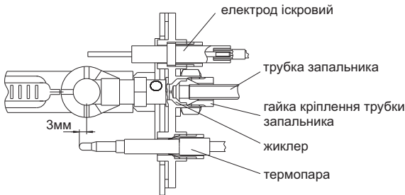
Рис. 3. Запальний пальник
